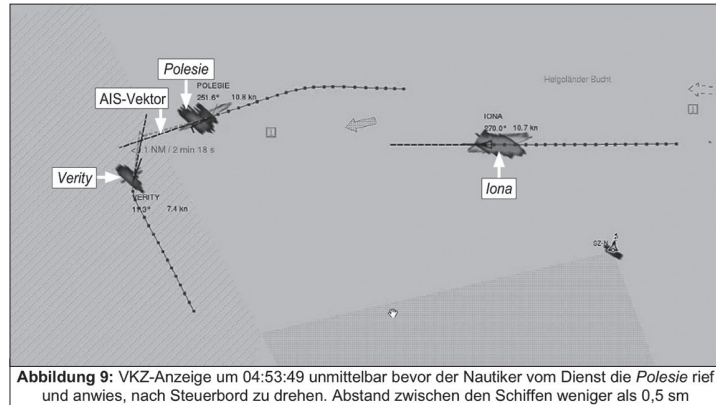
Abbildung 9: VKZ-Anzeige um 04:53:49 unmittelbar bevor der Nautiker vom Dienst die Polesie rief und anwies, nach Steuerbord zu drehen. Abstand zwischen den Schiffen weniger als 0,5 sm Der Routenverlauf kurz vor der Kollision von „Verity“ und „Polesie“.
