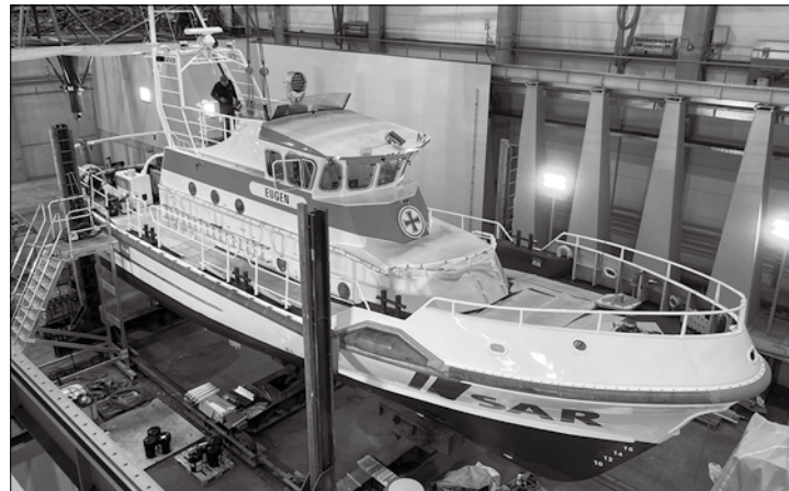
Lackiert und wieder mit Namensschildern glänzt die Eugen auf ihrem Platz in der Rostocker Werft. Foto: DGzRS
